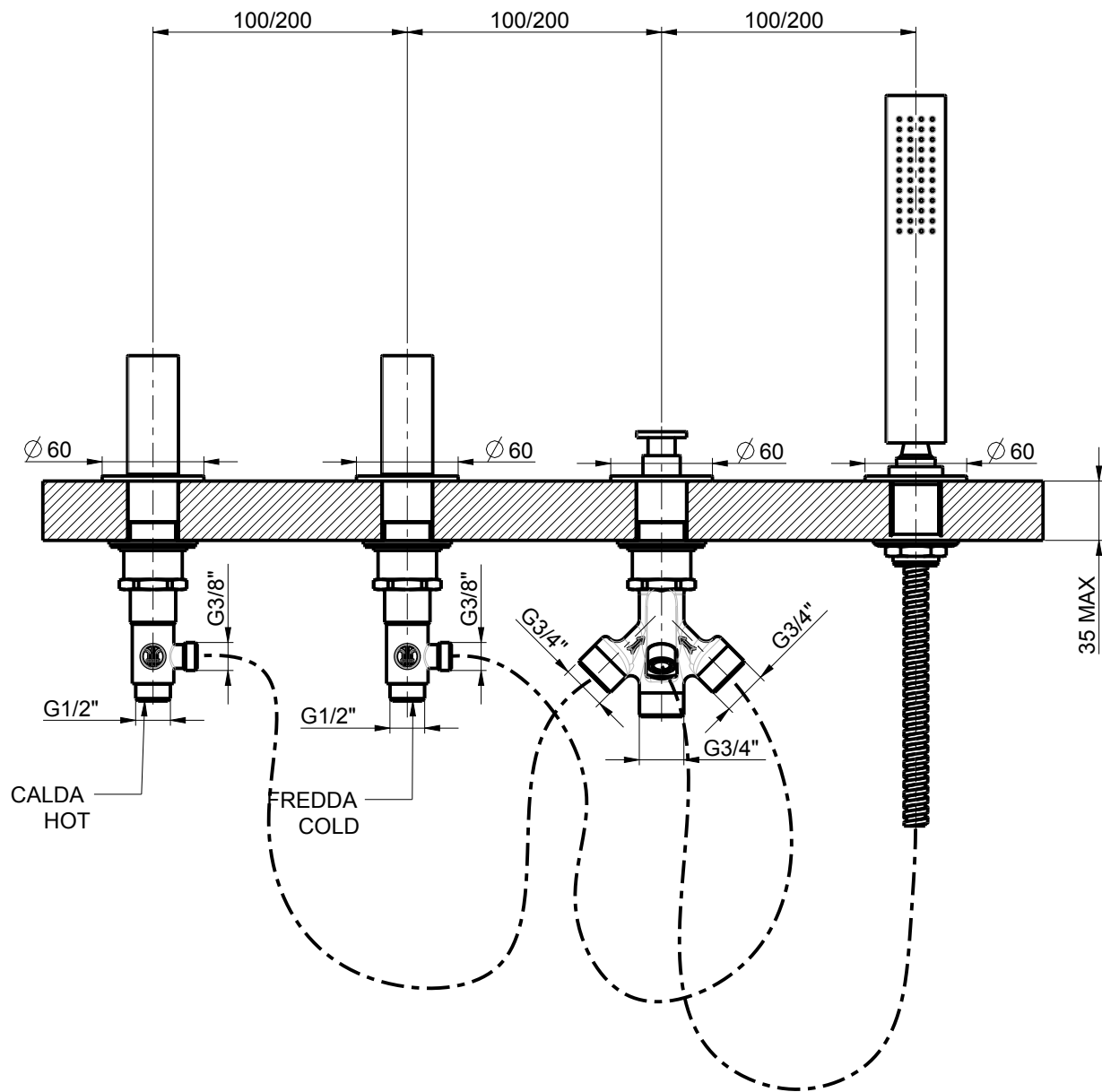
- Schema di foratura consigliato / Recommended drilling scheme
